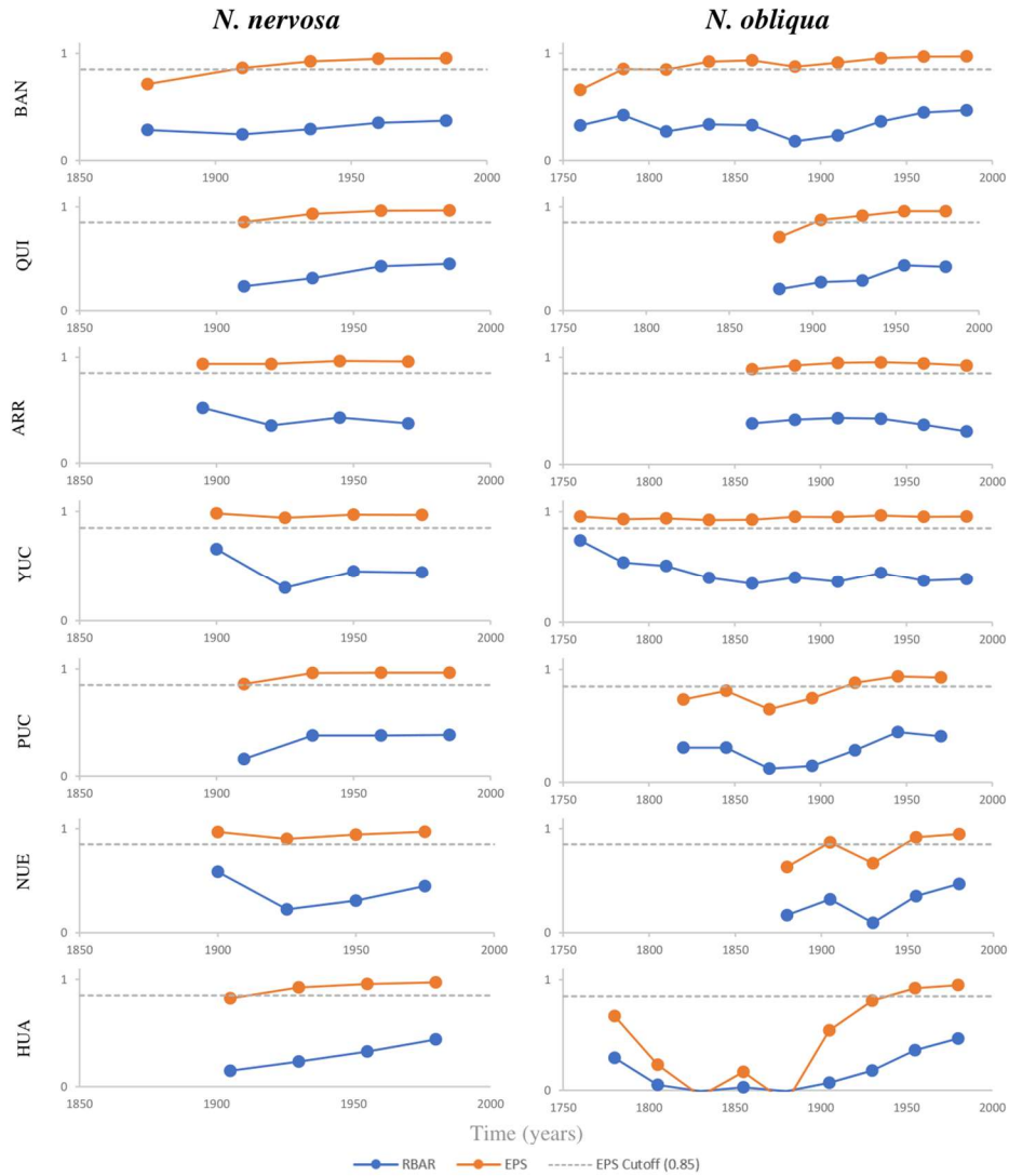
Fig. S1. Running EPS and RBAR for N. nervosa and N. obliqua chronologies.
